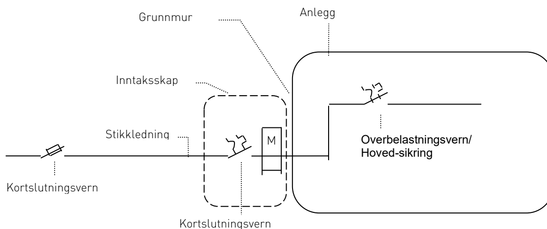
Figur 1 Eksempel på utvendig plassert målerskap
